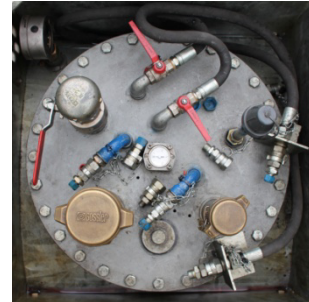
Draufsicht Domdeckel mit Anschlüssen
