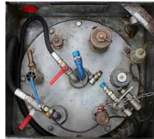
Draufsicht Domdeckel mit Anschlüssen
