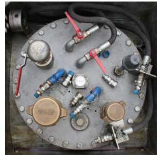
Draufsicht Domdeckel mit Anschlüssen
